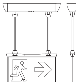
Velos + 48cm (ISO30061) (O-ESA-PS30) cijevni ovjes
