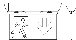
Jedinica napajanja + znak za izlaz → Velos
